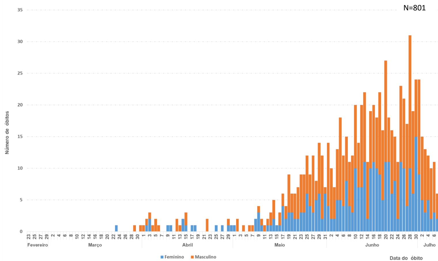
Figura 2. Curva dos óbitos confirmados de COVID-19 notificados no DF, segundo a data de ocorrência do óbito, 8 de julho de 2020.
