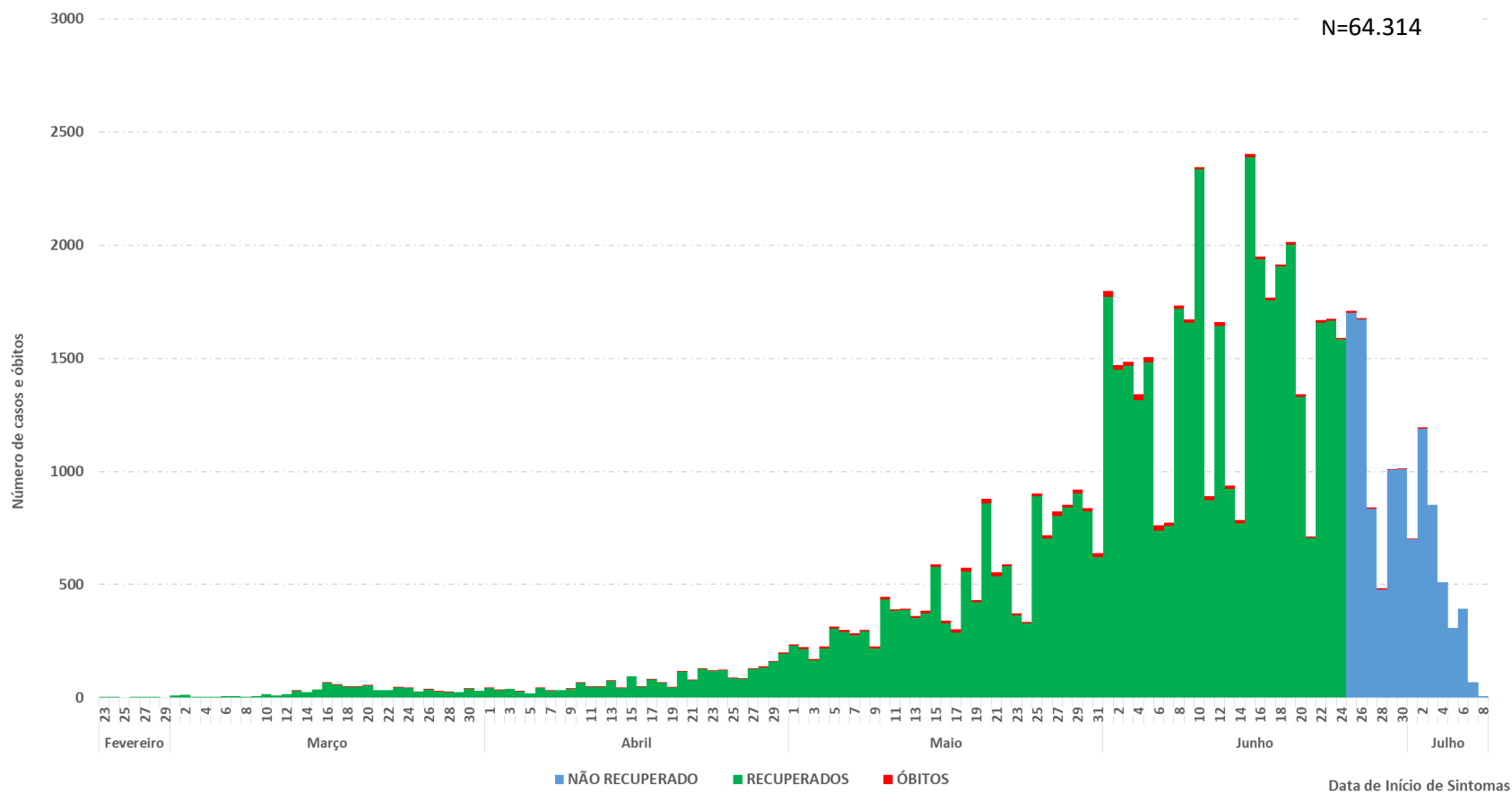
Figura 1. Curva epidemiológica dos casos confirmados de COVID-19 segundo evolução e data de início de sintomas. DF, 8 de julho de 2020.
